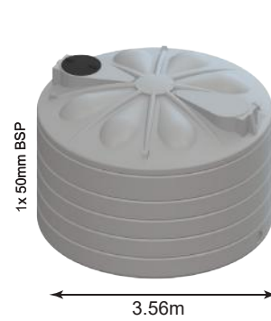
AQ21000 (21,036 ltrs)
